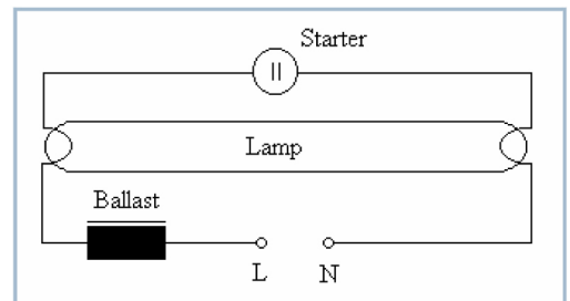
Схема включения
